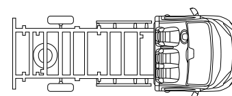
Leiterrahmen L4
